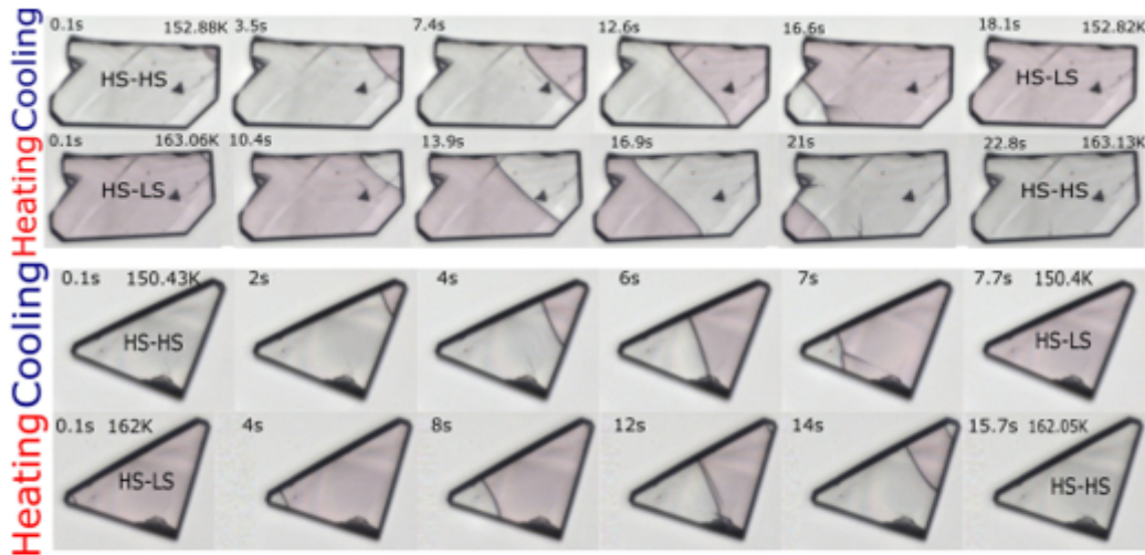
Fig1 : Observation sous microscope optique de la transition de cristaux à transition de spin en fonction de la température
